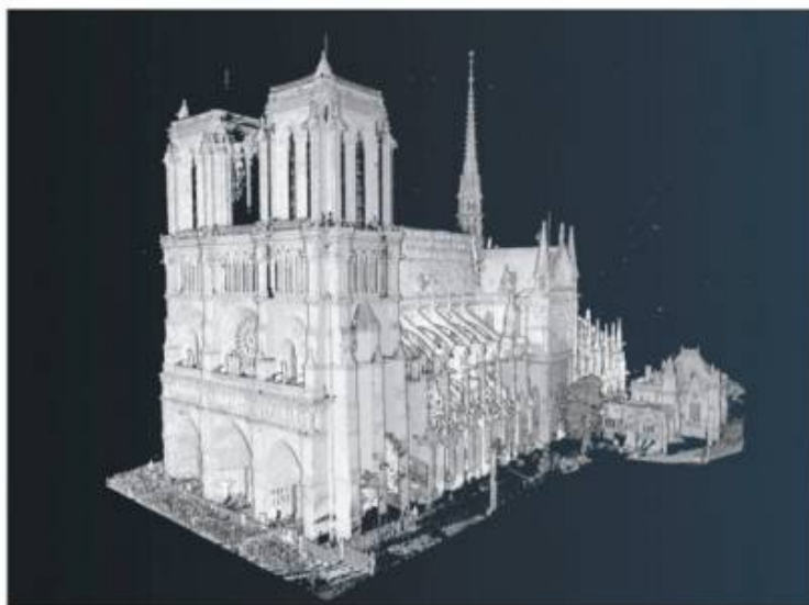
Nuage de points 3D, de la face sud-ouest de la cathédrale Notre-Dame de Paris, issu des campagnes de relevé.
